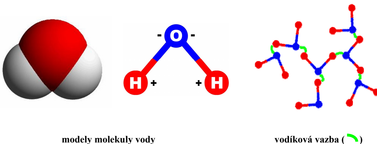
Obr. 2 Modely molekuly vody a vodíkové vazby
