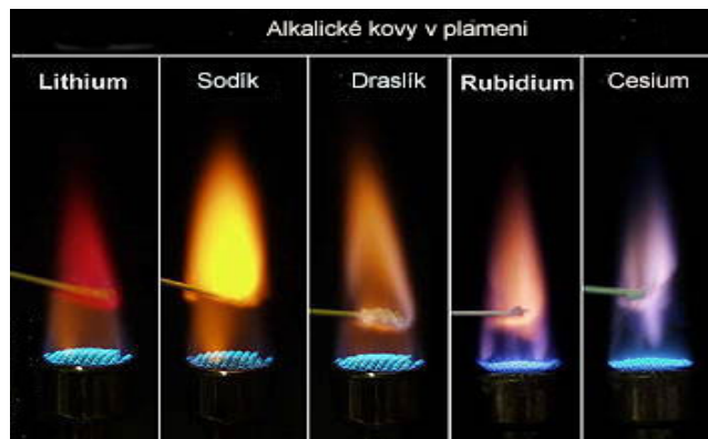
Obr. 5 Vlastnosti alkalických kovů
