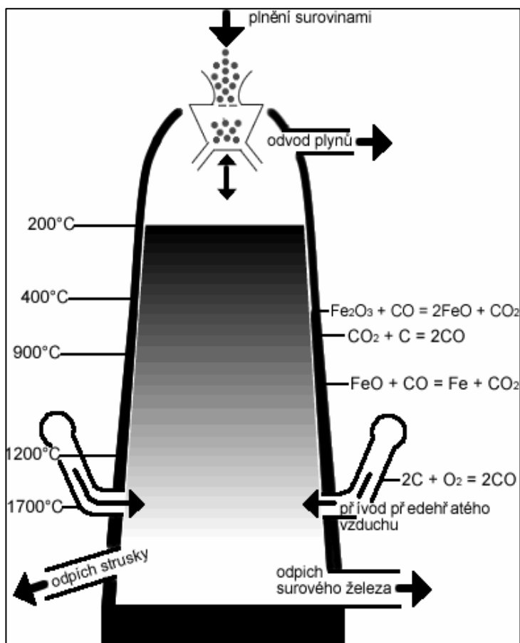
Obr. 7. Vysoká pec
