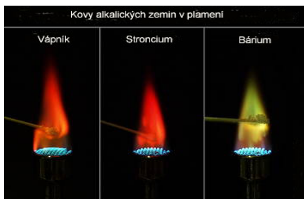
Obr. 6 Reakce prvků alkalických zemin v plameni
