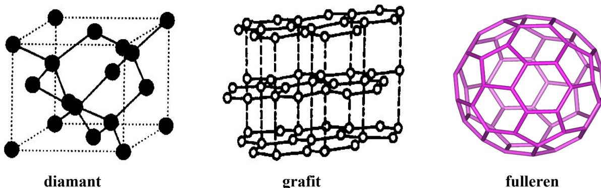
Obr. 3 Struktura alotropických modifikací uhlíku
